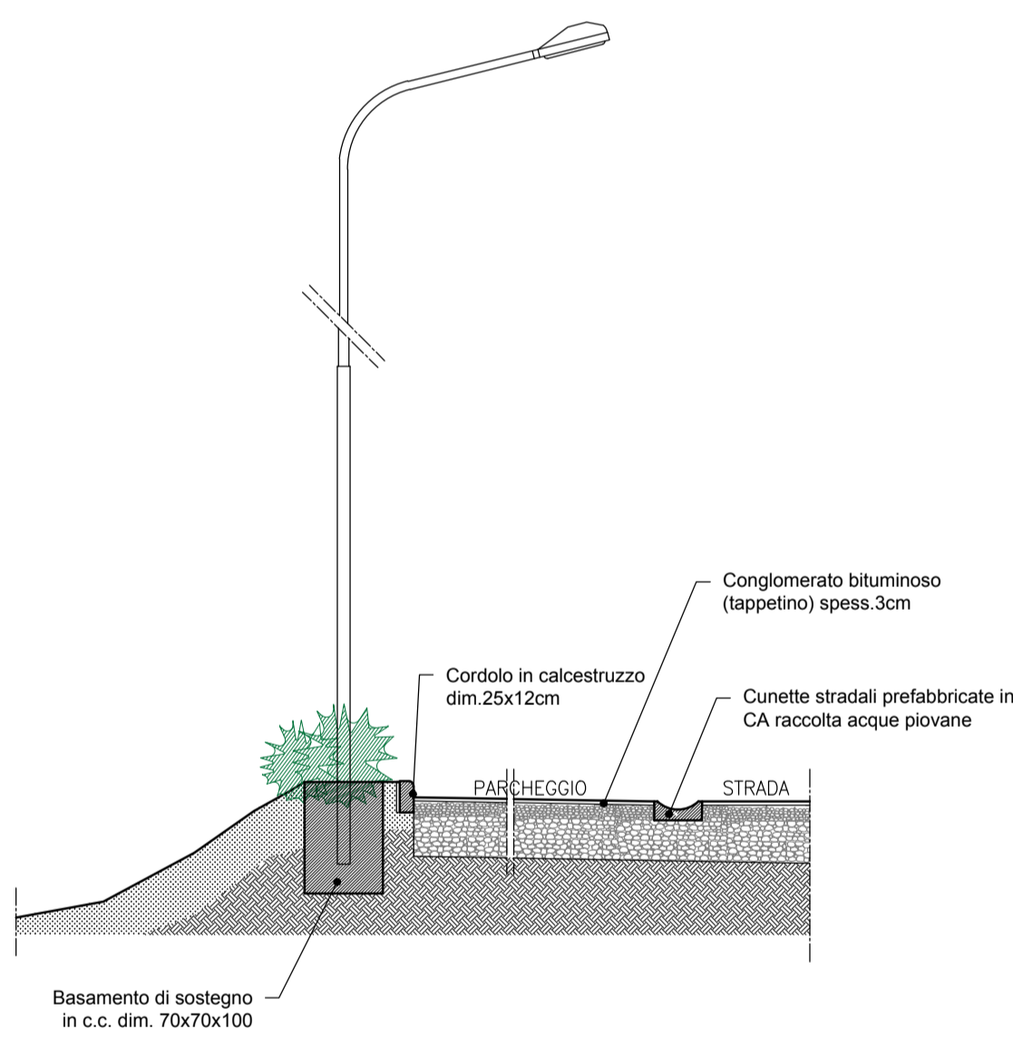
PARTICOLARE ESECUTIVO d.1 delle aree da cedere scala 1:50
